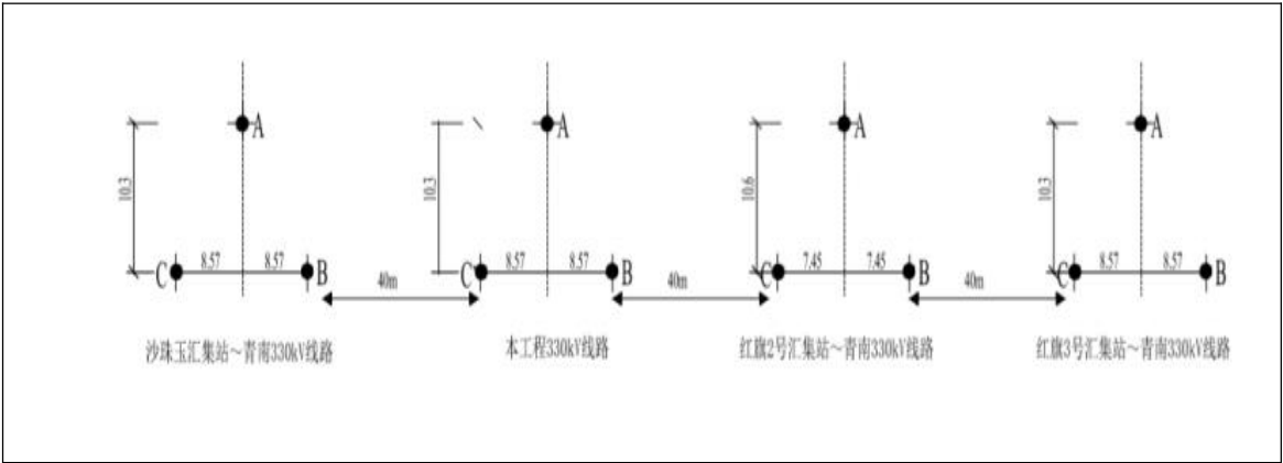
图 4-3 本工程线路与其他并行线路纵断面示意图
